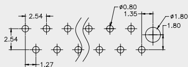
Recommended P.C.B Layout( Top Side)
